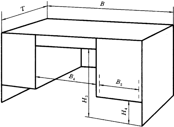
图 8 双柜桌尺寸示意图
