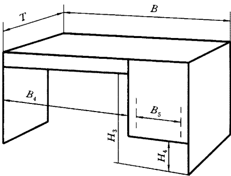
图 9 单柜桌尺寸示意图
