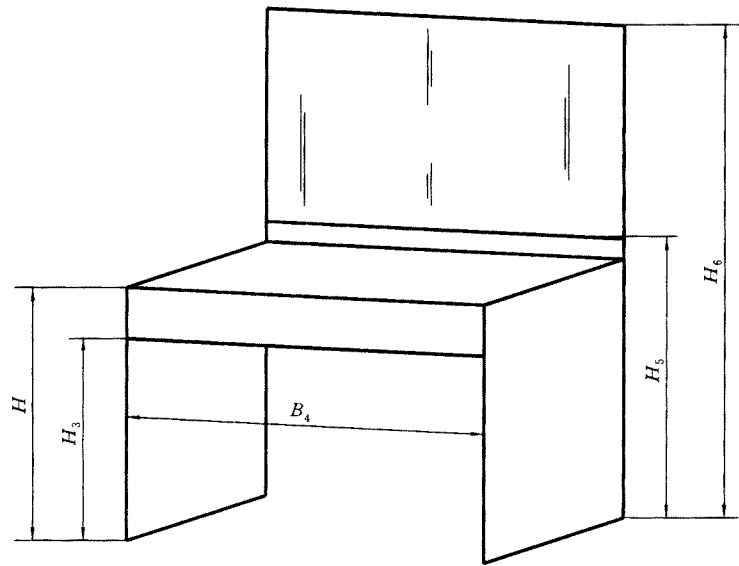
图 11 梳妆桌尺寸示意图
